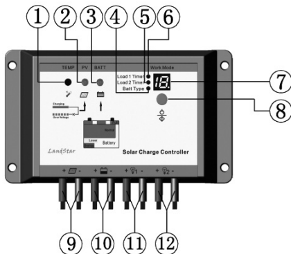
Rys. 2.1 Widok ogólny
