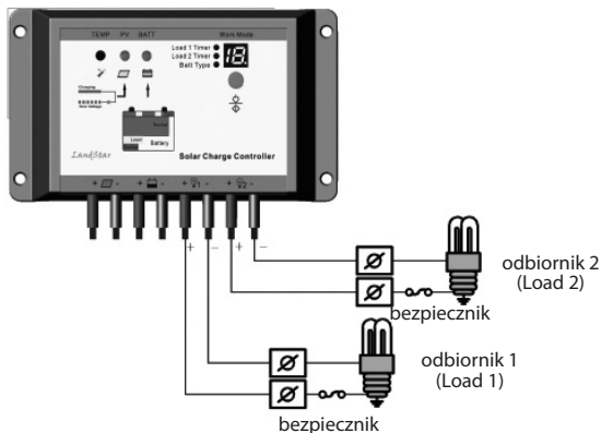
Rys. 3.3 Podłączenie odbiornika
