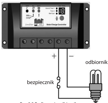
Rys. 3.3 Podłączenie odbiornika
