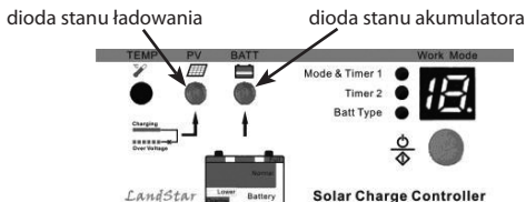
Rys. 4.2 Wskaźniki LED
