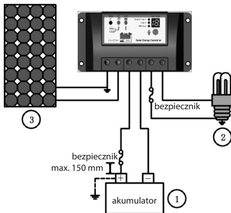
Rys. 3.4 Schemat połączeń całego układu
